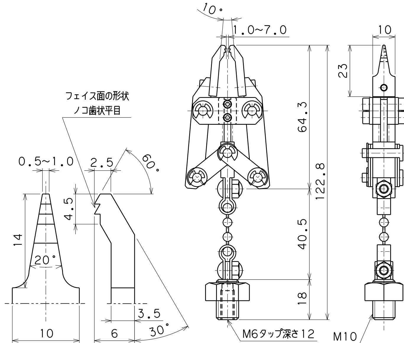
爪部拡大図 (S=3/1)
