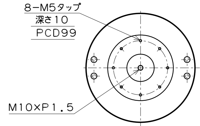
試料テーブル平面図
