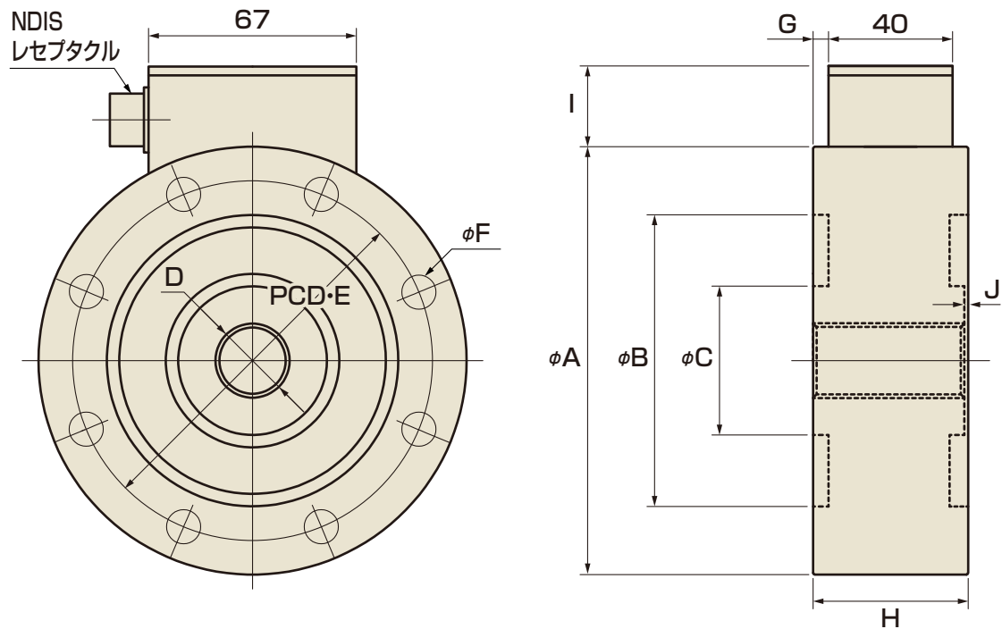
標準寸法表
