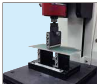
基板曲げ試験
