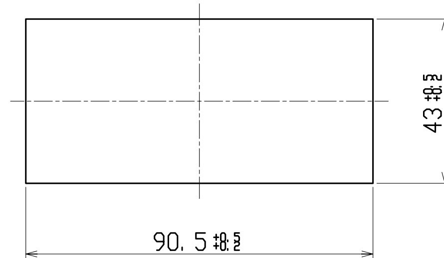
パネル取付用抜き穴寸法
